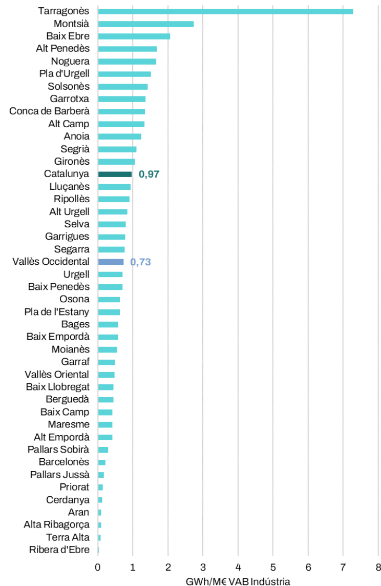
Gràfic 28. Intensitat energètica de la indústria (GWh/M€ VAB Indústria). Comarques de Catalunya. 2023
