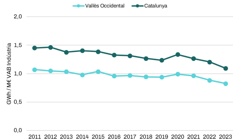
Gràfic 30. Evolució de la intensitat energètica de la indústria a preus constants (GWh/M€ VAB indústria). Vallès Occidental i Catalunya. 2011-2023
